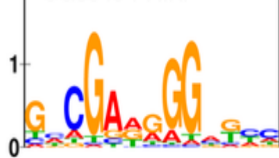
CG3340-PA:Kr
